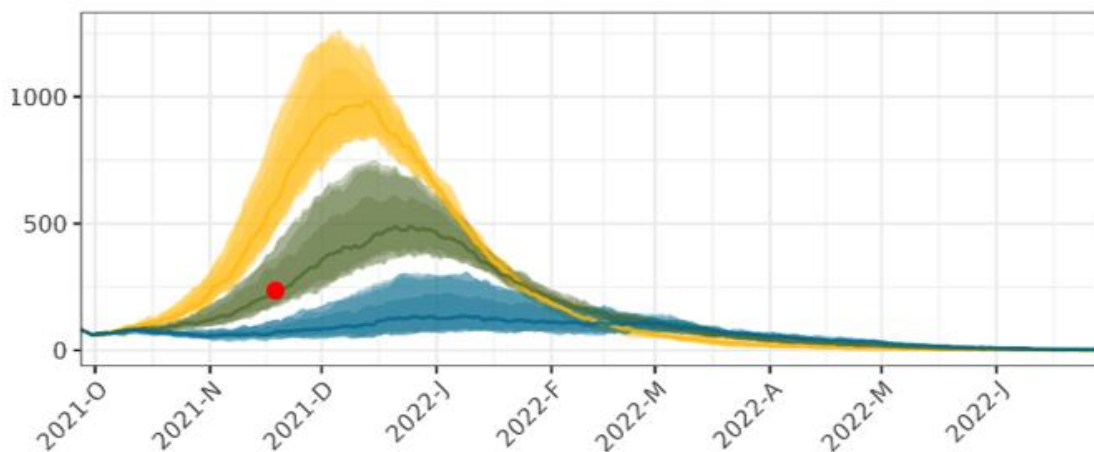
Figur 17. Antall daglig innleggelser på sykehus i perioden oktober 2021 – juni 2022 i et scenario med 90 % vaksinasjonsdekning, 50 % etterlevelse av selv-isolering, 25 % sesongeffekt og R_e på 1,1 (blå linje), 1,3 (grønn linje) eller 1,5, (gul linje).
