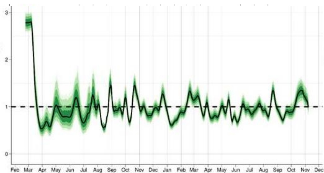
Figur 14. Anslag over det effektive reproduksjonstallet R_e i Norge fra februar 2020 til november 2021. Dataene er fra Folkehelseinstituttets jevnlig modellering av epidemien.
