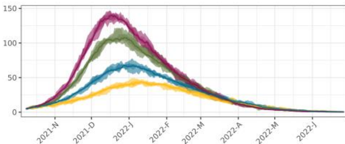
Figur 16. Antall daglig innleggelser på sykehus i perioden oktober 2021 – juni 2022 i et scenario med 90 % vaksinasjonsdekning hos alle over 12 år, 25 % sesongeffekt, R_0 6,0 og varierende grad av etterlevelse av selvisolering. Rød linje er 0 % etterlevelse, grønn linje er 20 % etterlevelse, blå linje er 50 % etterlevelse og gul linje er 70 % etterlevelse.
